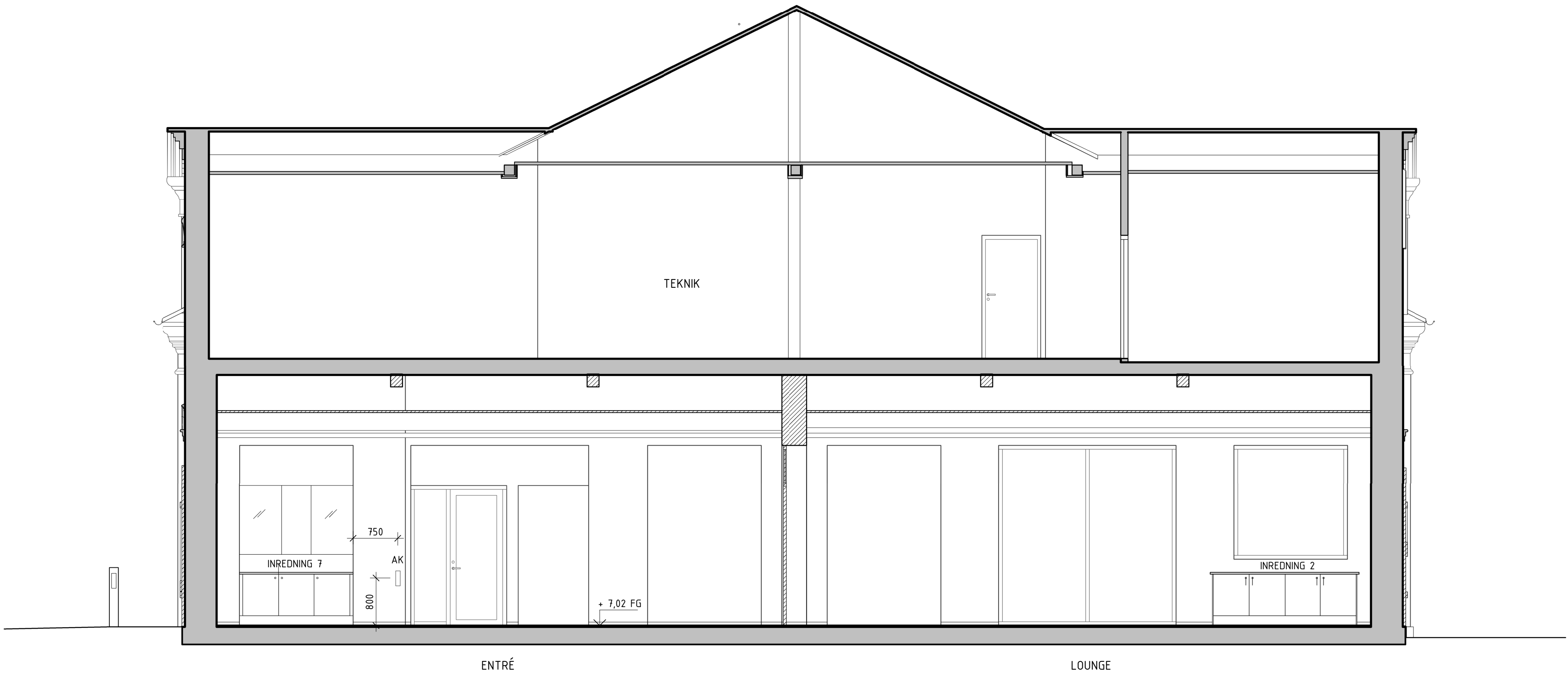
SEKTION C-C
