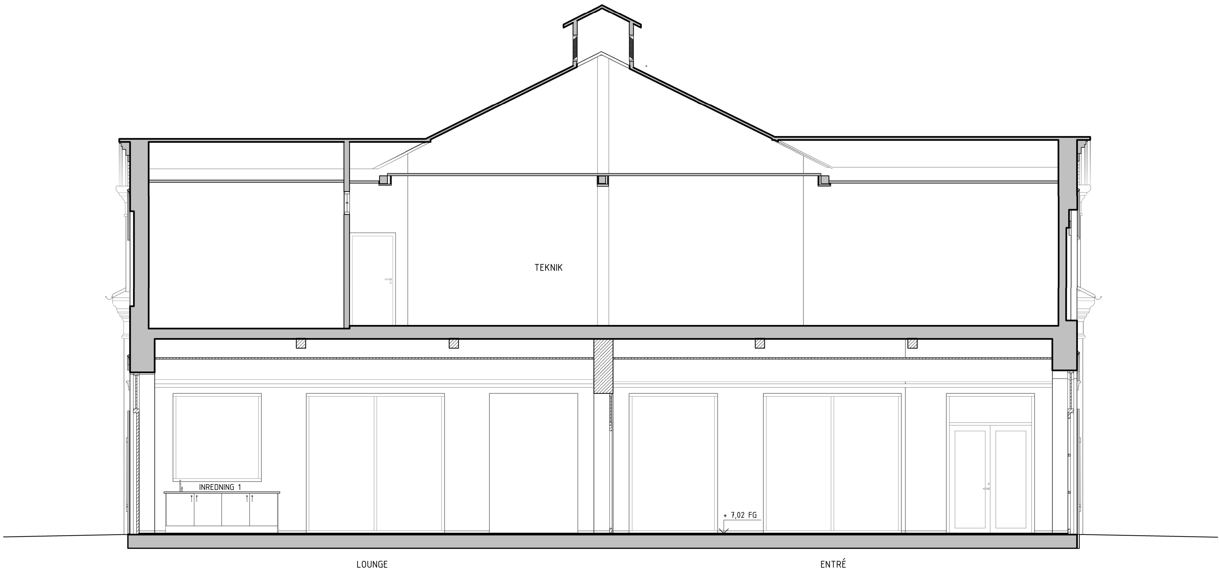
SEKTION B-B
